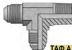
ΤΑΦ Α. UNF- Α. UNF- Α. NPT
