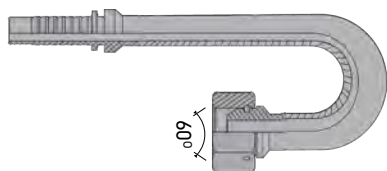
ΓΩΝΙΑ BSP 180°
