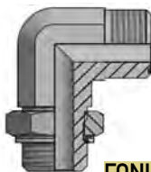
ΓΩΝΙΑ 90° O.R.F.S - ΒΑΣΗ BSP
