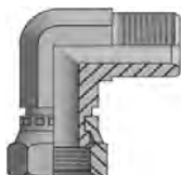
ΓΩΝΙΑ ΑΡΣ. - ΘΗΛ. BSP
