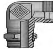
ΓΩΝΙΑ 90° ΜΕ ΒΑΣΗ UNF ΚΟΝΤΡΑ
