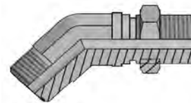
ΓΩΝΙΑ 45° ΚΟΝΤΡΑ O.R.F.S.
