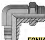
ΓΩΝΙΑ 90° ΑΡΣ. UNF - ΑΡΣ. UNF ΒΑΣΗ
