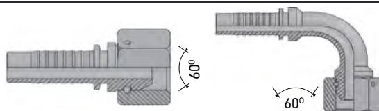
BSP 45° - 45H ΜΕ ΓΚΑΒΙΛΙΑ
