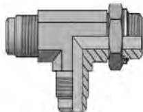
ΤΑΦ UNF ΑΡΣ. ΑΚΡΗ ΒΑΣΗ UNF
