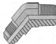
ΓΩΝΙΑ 45° ΑΡΣ. UNF - ΑΡΣ. NPT ΒΑΣΗ
