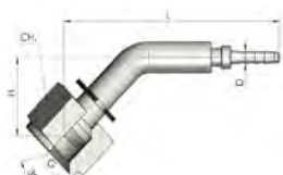
ΓΩΝΙΑ 45° INTΣΑΣ BSP S2
