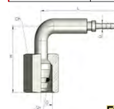
ΓΩΝΙΑ 90° ΜΑΝ/ΤΡΟΥ S2
