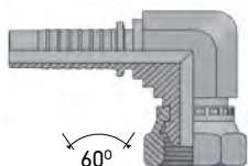
ΓΩΝΙΕΣ 90° BSP COMPACT
