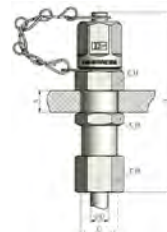
ΒΑΛΒΙΔΑ 16x2 ΘΗΛ. ΠΕΡ/ΦΟΜΕΝΟ O.R.F.S
