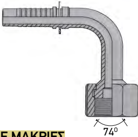
ΓΩΝΙΕΣ 90° UNF ΜΑΚΡΙΕΣ
