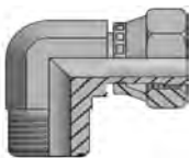
ΓΩΝΙΑ 90° O.R.F.S ΑΡΣ.-ΘΗΛ.
