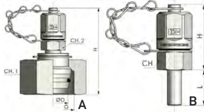
(Α) ΒΑΛΒΙΔΑ ΑΡΣ. 16x2 - ΘΗΛ. ΜΕΤΡ.
