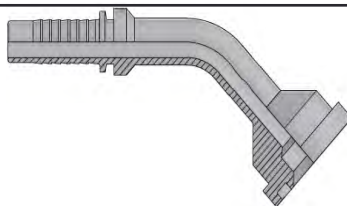
6000 PSI ΓΩΝΙΕΣ 45° ΜΑΚΡΥ ΣΤΕΛΕΧΟΣ
