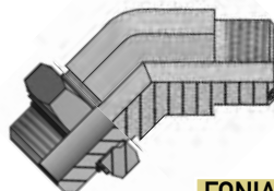
ΓΩΝΙΑ 45° O.R.F.S. - ΒΑΣΗ UNF
