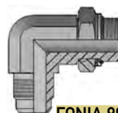
ΓΩΝΙΑ 90° ΑΡΣ. UNF-ΑΡΣ. ΜΕΤΡ. ΒΑΣΗ
