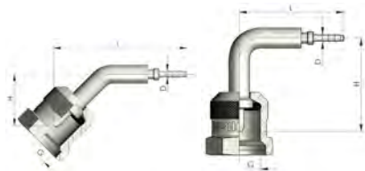
ΡΑΚΟΡ ΒΑΛΒΙΔΑΣ S2
