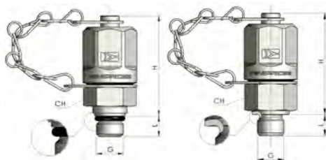
ΒΑΛΒΙΔΑ ΑΡΣ. 16x2 - ΑΡΣ. ΒΑΣΗ
