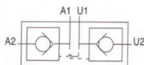
ΒΑΛΒΙΔΑ ΔΙΠΛΟΥ ΚΛΕΙΔΩΜΑΤΟΣ ΓΡΑΜΜΗΣ
