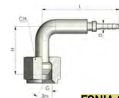
ΓΩΝΙΑ 90° INTΣΑΣ BSP S2
