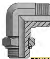
ΓΩΝΙΑ 90° O.R.F.S - ΒΑΣΗ ΜΕΤΡΙΚΟ
