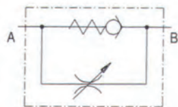
ΣΤΡΑΓΓΑΛΙΣΤΗΣ ΡΟΗΣ ΧΕΙΡΟΒΟΜΒΙΔΑ ΜΕ ΑΝΤΕΠΙΣΤΡΟΦΗ ΒΑΛΒΙΔΑ
