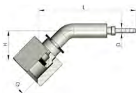
ΓΩΝΙΑ 45° ΜΑΝ/ΤΡΟΥ S2
