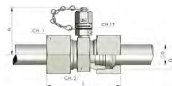
ΒΑΛΒΙΔΑ ΣΥΝΔΕΣΜΟΣ L - S
