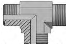
ΤΑΦ O.R.F.S A - A - A
